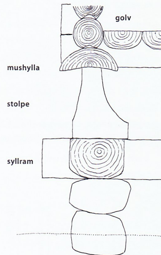
Grundläggning av härbren och magasin. I syllramens hörn står stolpar som syllen ligger på. Syllen består ofta av en halv stock som ligger med bredsida ner. Den kallas mushylla för att den hindrar möss och andra smådjur från att ta sig in.
